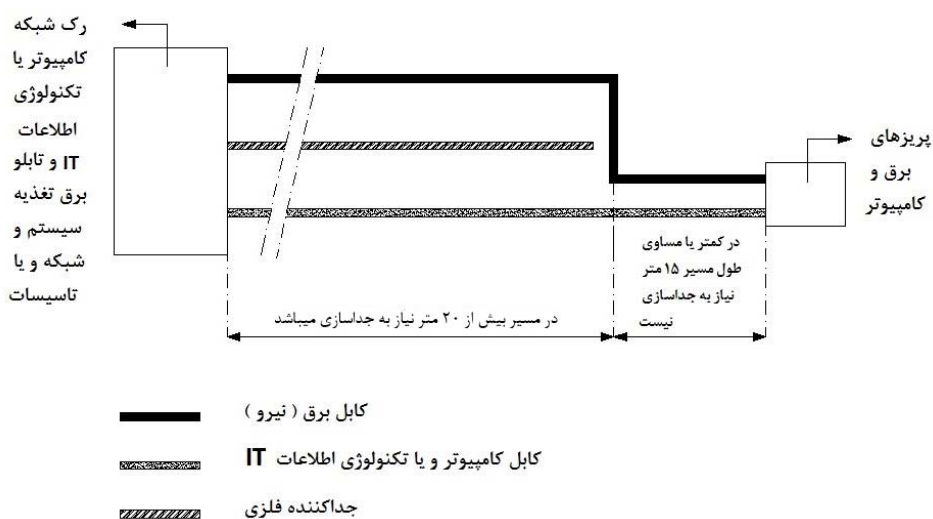
شکل ۱۳-۳-۲: ۲-۱۸-۱-۳: طرحواره مسیر مجزا و مشترک کابل برق و کابل کامپیوتر یا فناوری اطلاعات IT برای طول مسیر بیش از ۳۵ متر
