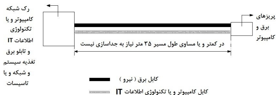
شکل ۱۳-۳-۱: ۱-۱۸-۱-۳: طرحواره مسیر مشترک کابل برق و کابل کامپیوتر یا فناوری اطلاعات IT برای طول مسیر کمتر یا مساوی ۳۵ متر
