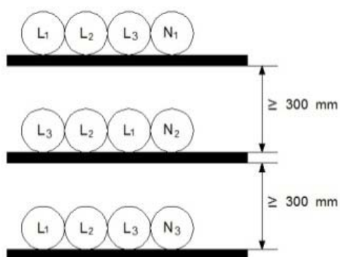
شکل ۷-۱۳-۱-۷-۱: آرایش چسبیده به هم در سه تراز و هر تراز به فاصله ۳۰ سانتی متر از هم برای رشته کابل تک رشته موازی (سه فاز)
